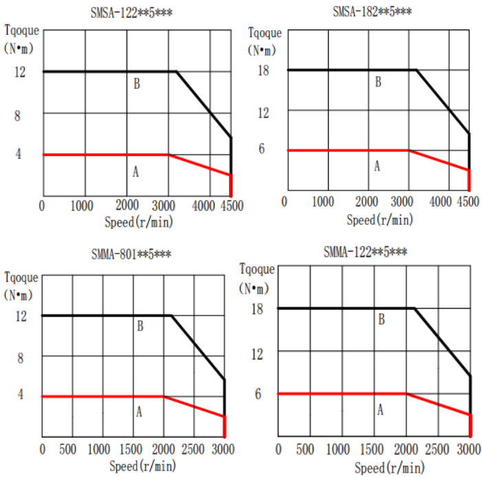
130 法兰伺服电机转矩-转速特性曲线
