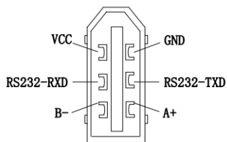
图 4.3.13 通讯口 CN1 插头端子排列顺序图
