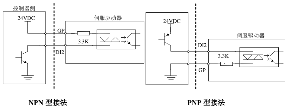
图 4.3.5 有源接点接口电路
