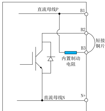
图 7.1.10 伺服内部能耗制动示意图
