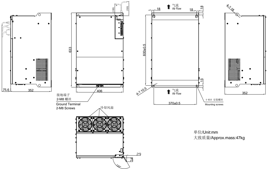
图 3.1.13 伺服驱动器结构尺寸 11
