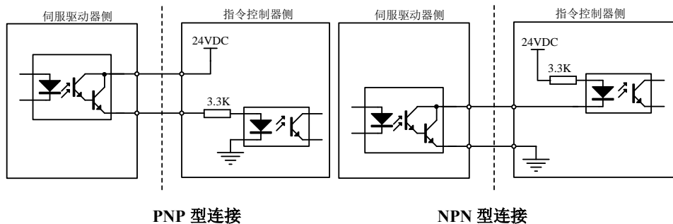
图 4.3.9 光电耦合器输出接口电路
