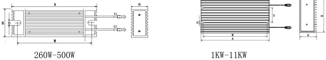
图 7.1.12 伺服铝壳制动电阻结构图
