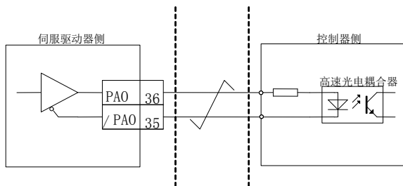
图 4.3.10 编码器分频输出的光电耦合器接口电路
